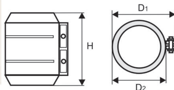
Rohrverbinder aus Edelstahl mit Brandschutzeigenschaften für Rohrsysteme aus Gussrohr nach DIN 19522/EN 877. Geprüft nach DIN EN 877.
