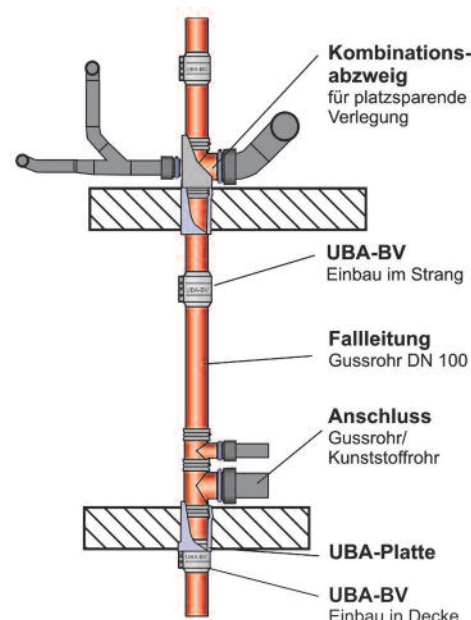
Bild 3 • Für den variablen Einbau: Der UBA-BV Brandschutzverbinder ist eine baustellengerechte Brandschutz-Lösung (mit abZ) für Mischinstallationen.
